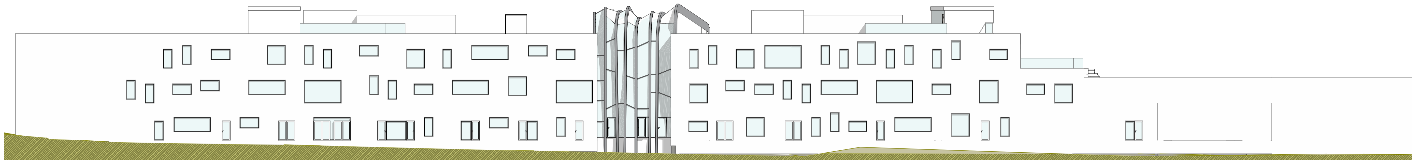
Vest 1:200
